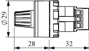
Montaj Ölçüsü Ø22.4 ±0.2 mm
